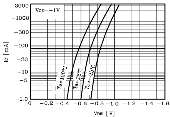
IC - V BE
