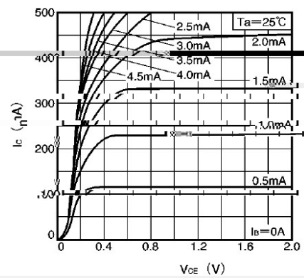
I_C - V_{CE}
