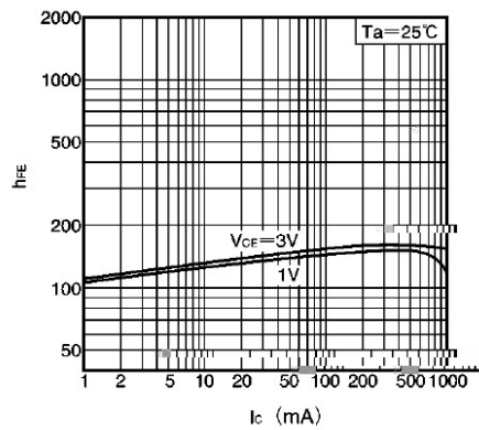
h_{FE} - I_C
