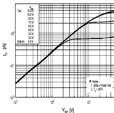
I_D - V_{DS}
