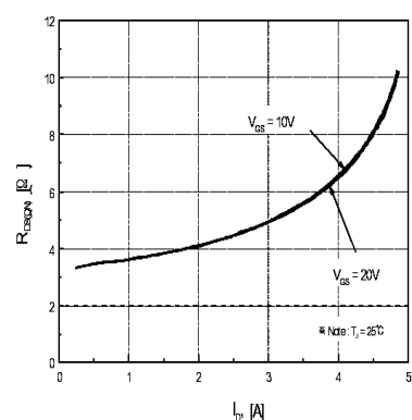
R_{DS(on)} - I_D
