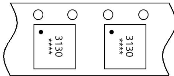
编带示意图
