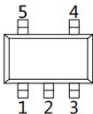
SOT23-5
