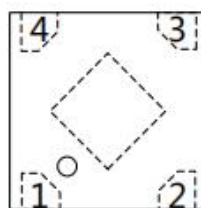
DFN1*1-4L
