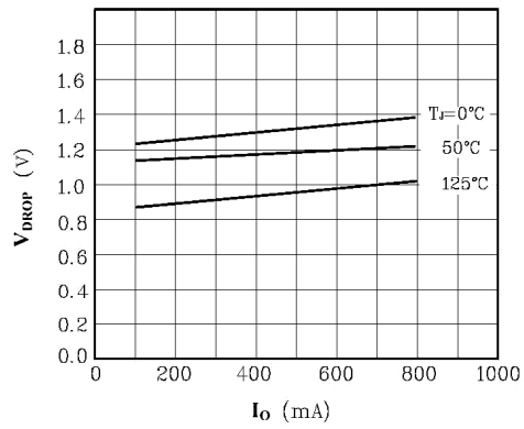
V_{DROP} - I_O
