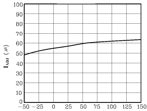
I_{ADJ} - T_a
