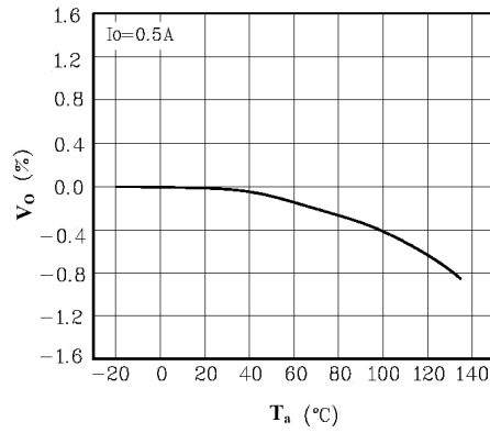
V_O - T_a
