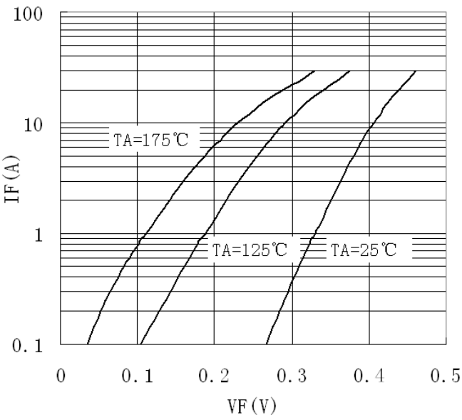
IF - VF
