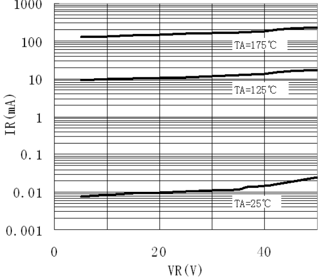
IR - VR
