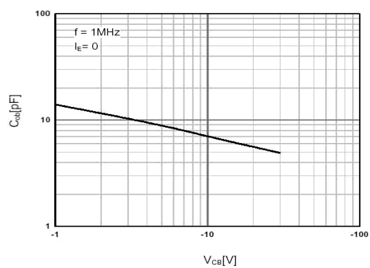
C_{ob} - V_{CB}
